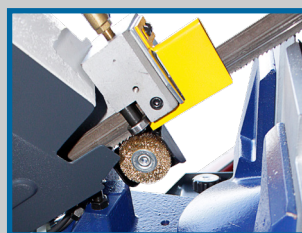
Patins carbure guide lame et brosse
