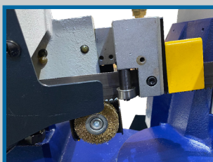
Patins carbure guide lame et brosse
