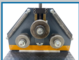
Galets supérieurs et inférieurs
