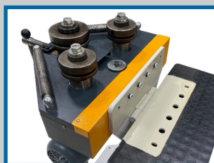
Tête inclinable
